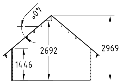
SEKTION
