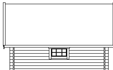
FASAD
