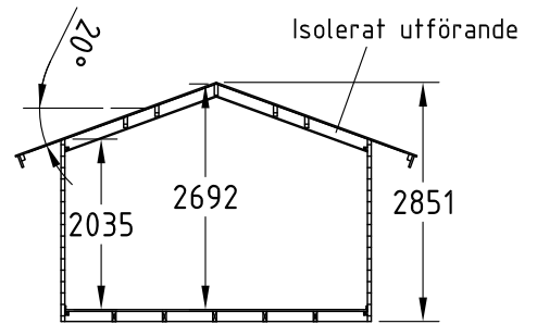
SEKTION
