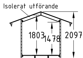
SEKTION
