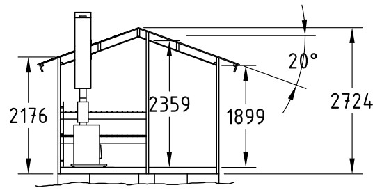
SEKTION
