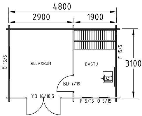
PLAN MED PARDÖRR
