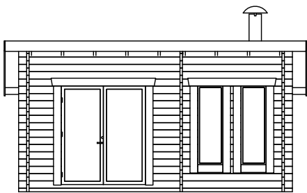
FASAD MED PARDÖRR
