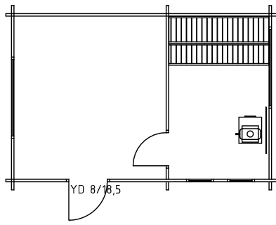
PLAN MED ENKELDÖRR
