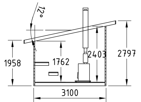
SEKTION
