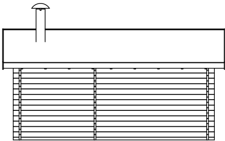
FASAD
