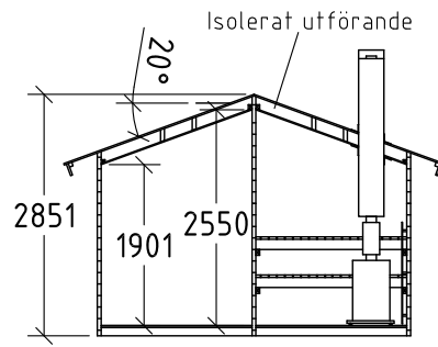
SEKTION
